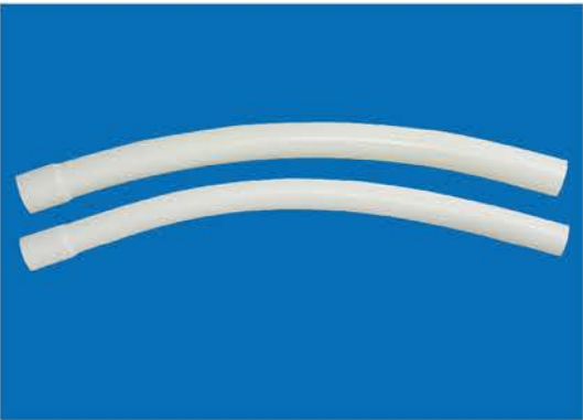
PVC 料线用弯管 编码: 21102、21109
